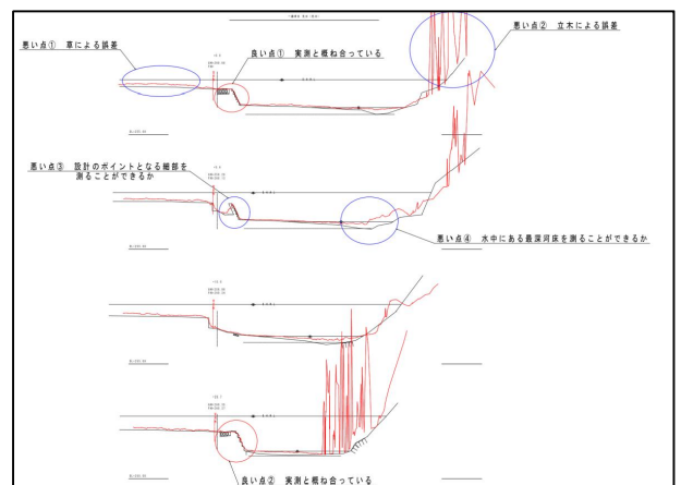
横断面図と実測横断面図との比較検証例
